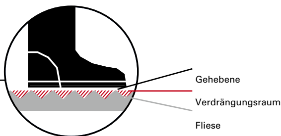
Der Verdrängungsraum ist der rot gekennzeichnete Hohlraum zwischen den Erhebungen der Fliese unterhalb der Gehebene
