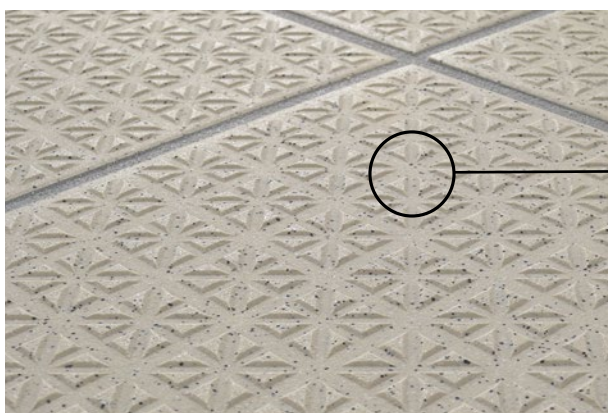
Der Verdrängungsraum ist der rot gekennzeichnete Hohlraum zwischen den Erhebungen der Fliese unterhalb der Gehebene
